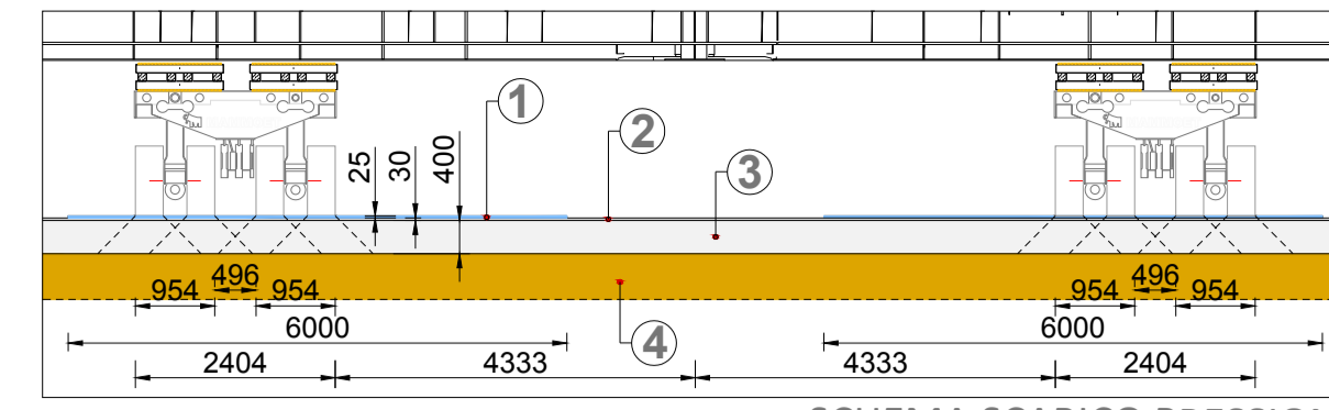
SCHEMA SCARICO PRESSIONI SISTEMA DI TRASPORTO
